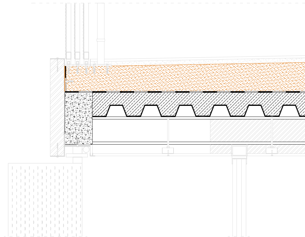
fase_4 getto del massetto delle pendenze (2%)
