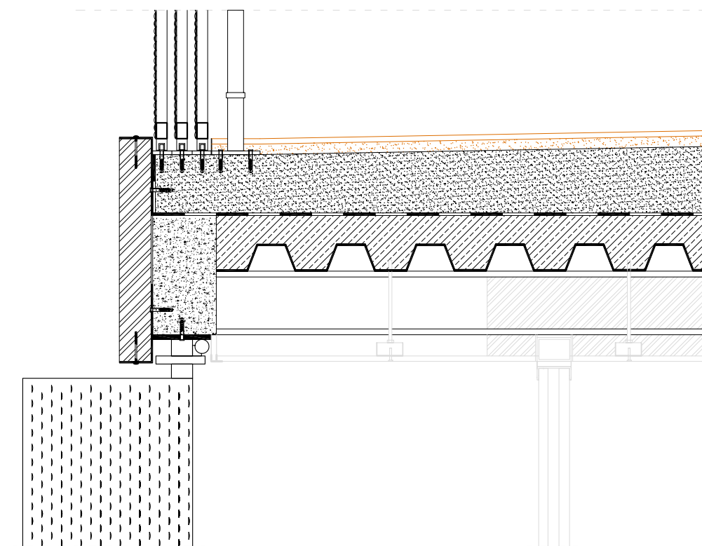
fase_7 stesura della malta di allettamento e posa della pavimentazione
