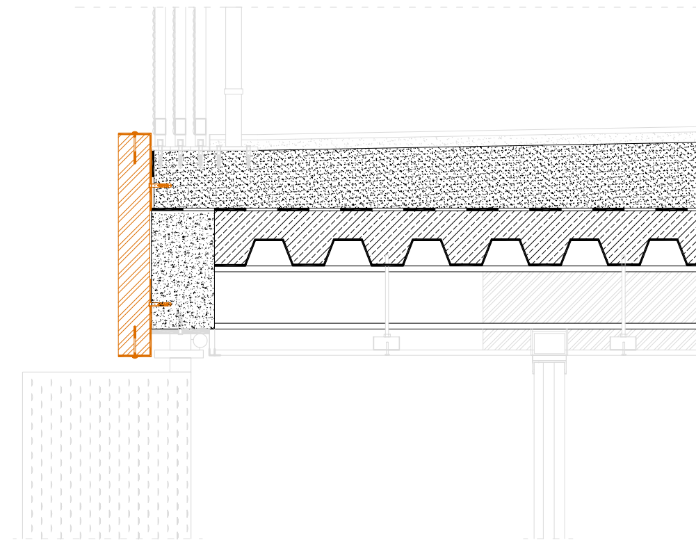
fase_5 posa del pannello in poliuretano espanso rigido rivestito in lamiera di alluminio
