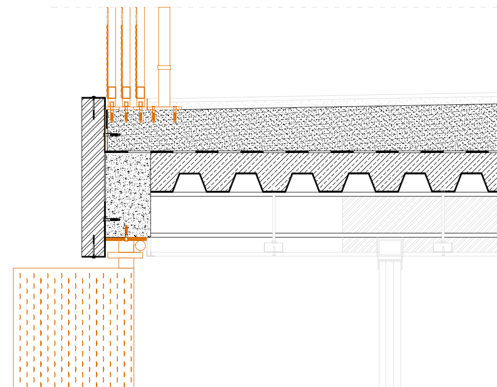
fase_6 montaggio dei pannelli scorrevoli, delle lamelle orientabili, del relativo sistema sincronizzato di movimentazione
